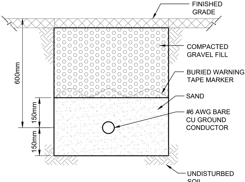
B GROUNDING TRENCH DETAIL SCALE: N.T.S.
