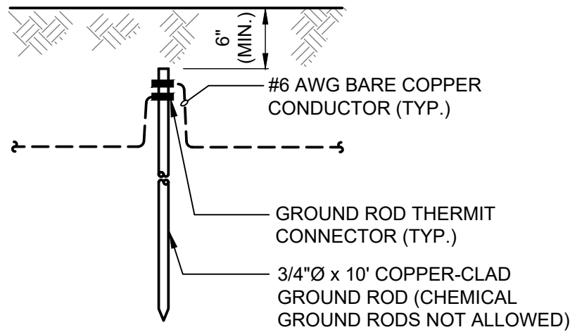
C GROUND ROD DETAIL SCALE: N.T.S.
