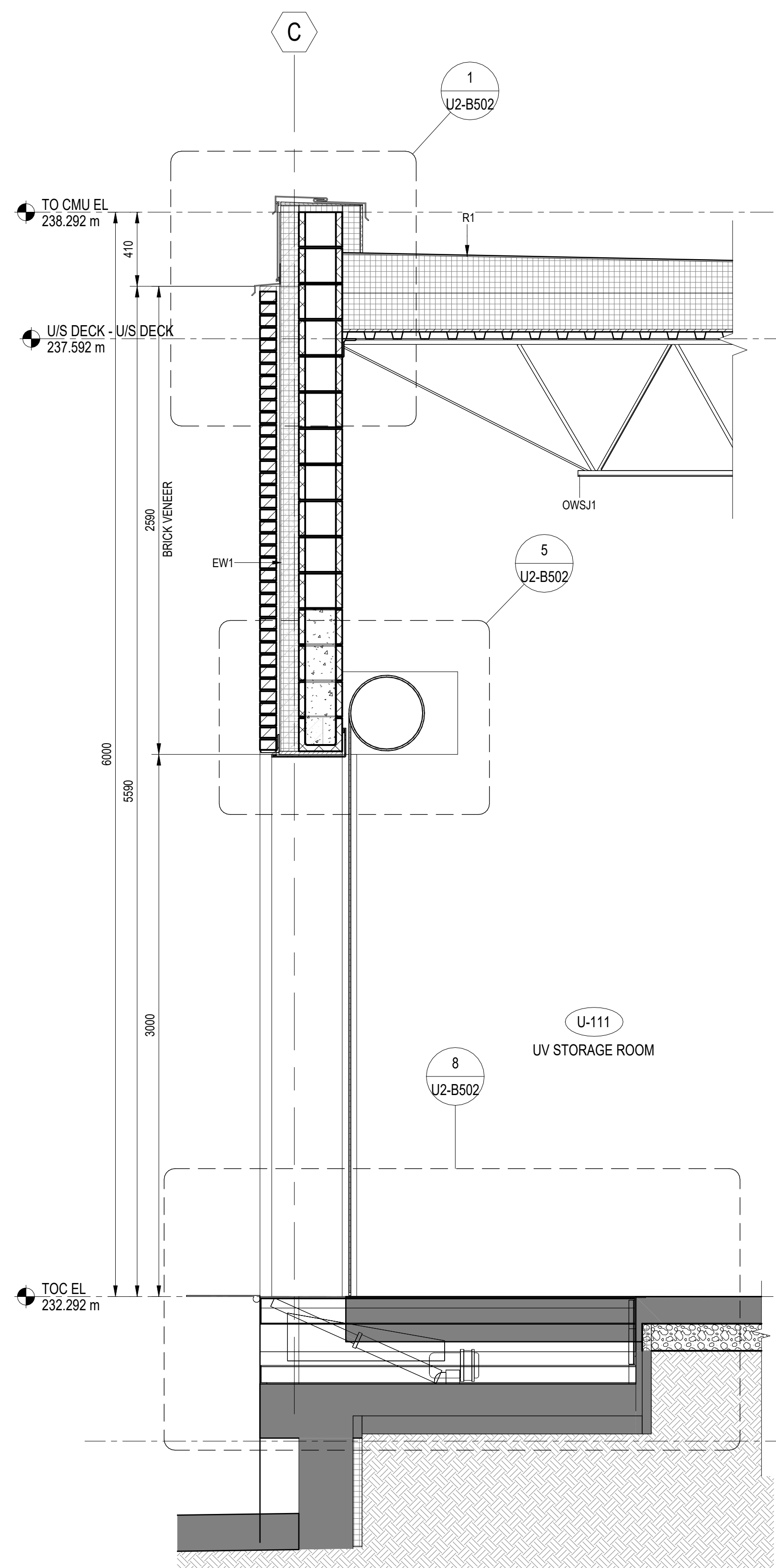
1 WALL SECTION - 1 U2-B201 SCALE: 1 : 20
