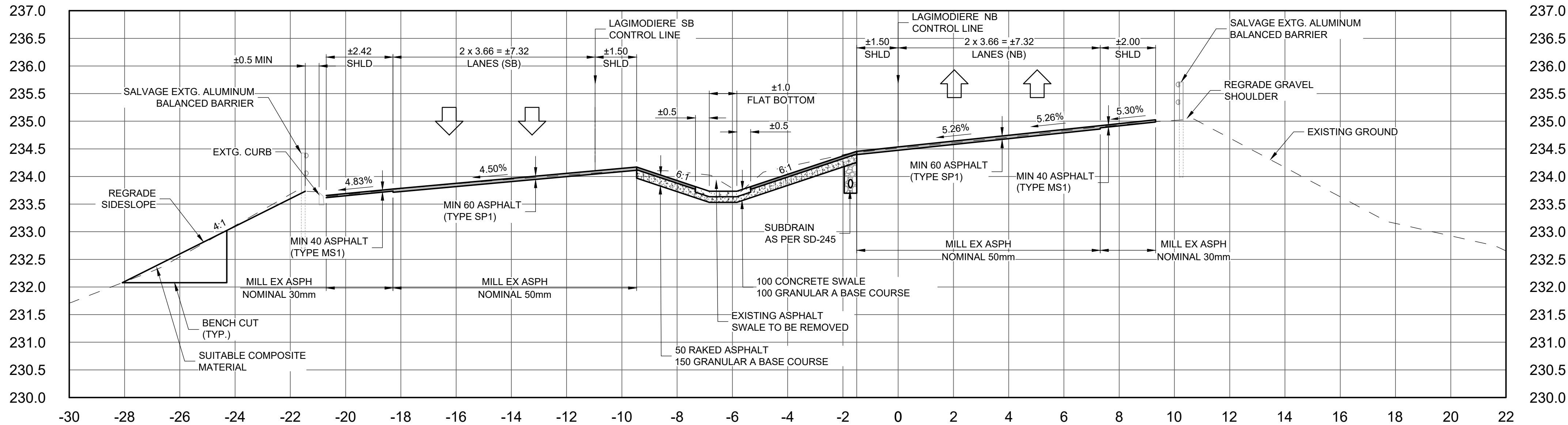
4 4209 4302 H 1:100, V 1:50 SECTION - STA 20+920 (NB)
