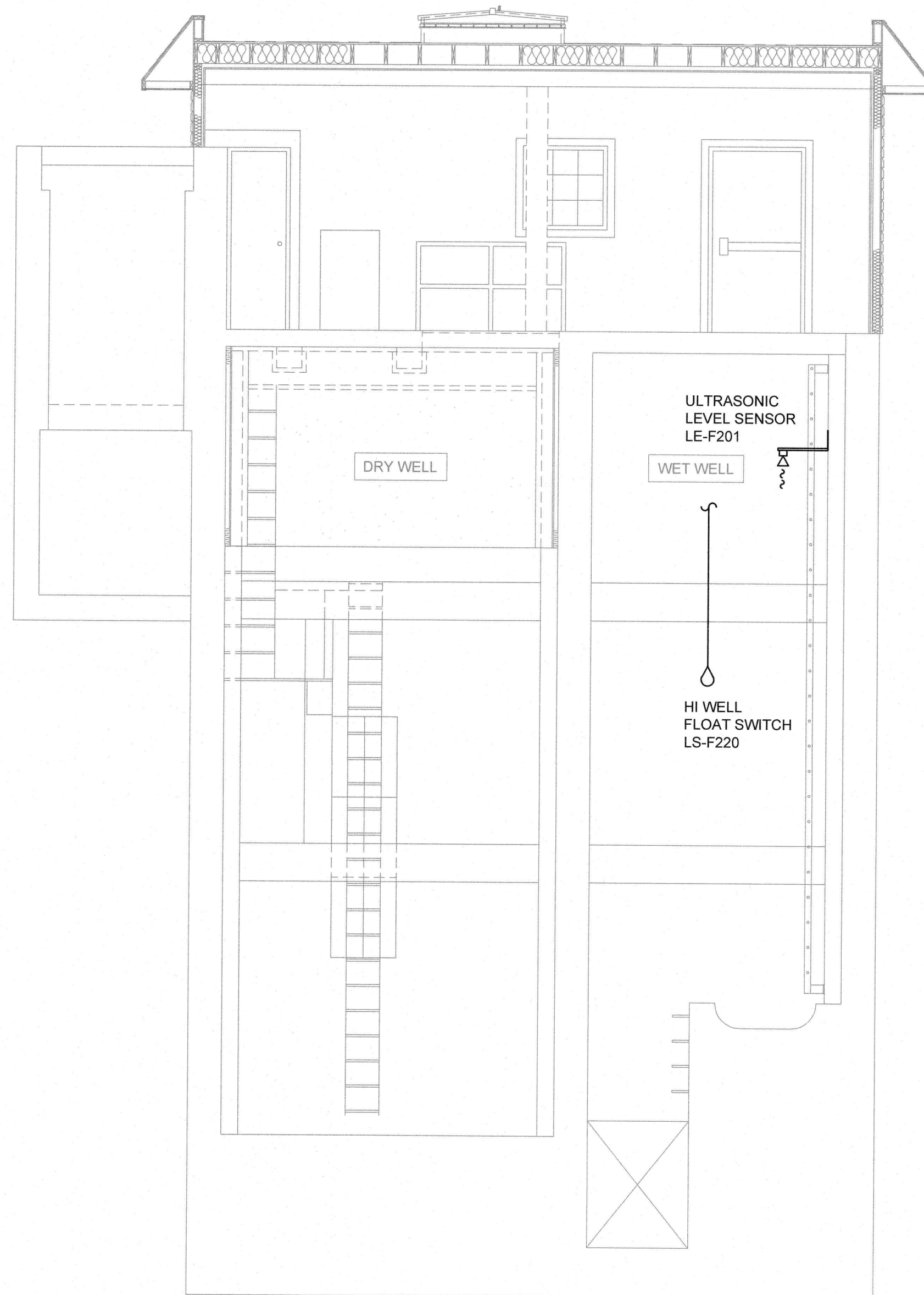
4 SECTION E0002 E0003 1:50
