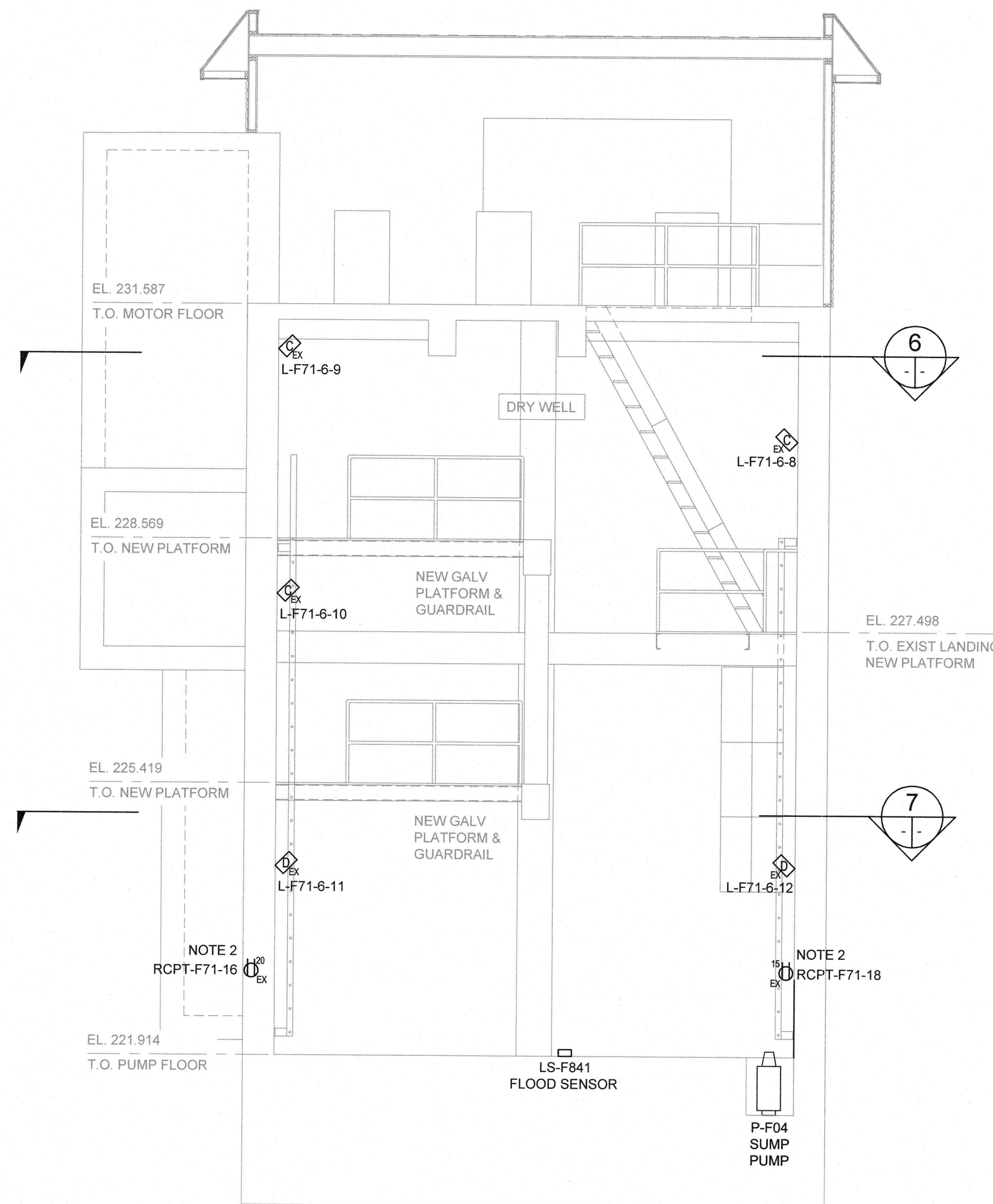
5 SECTION E0002 E0003 1:50
