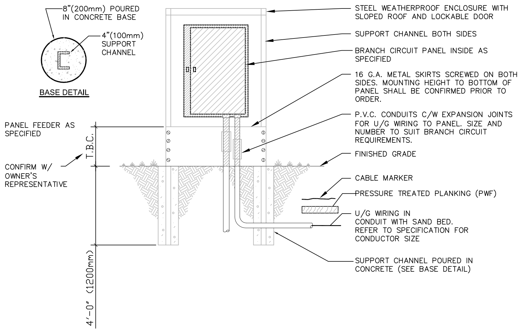
3 WEATHERPROOF PANELBOARD E1.0 SCALE: N.T.S
