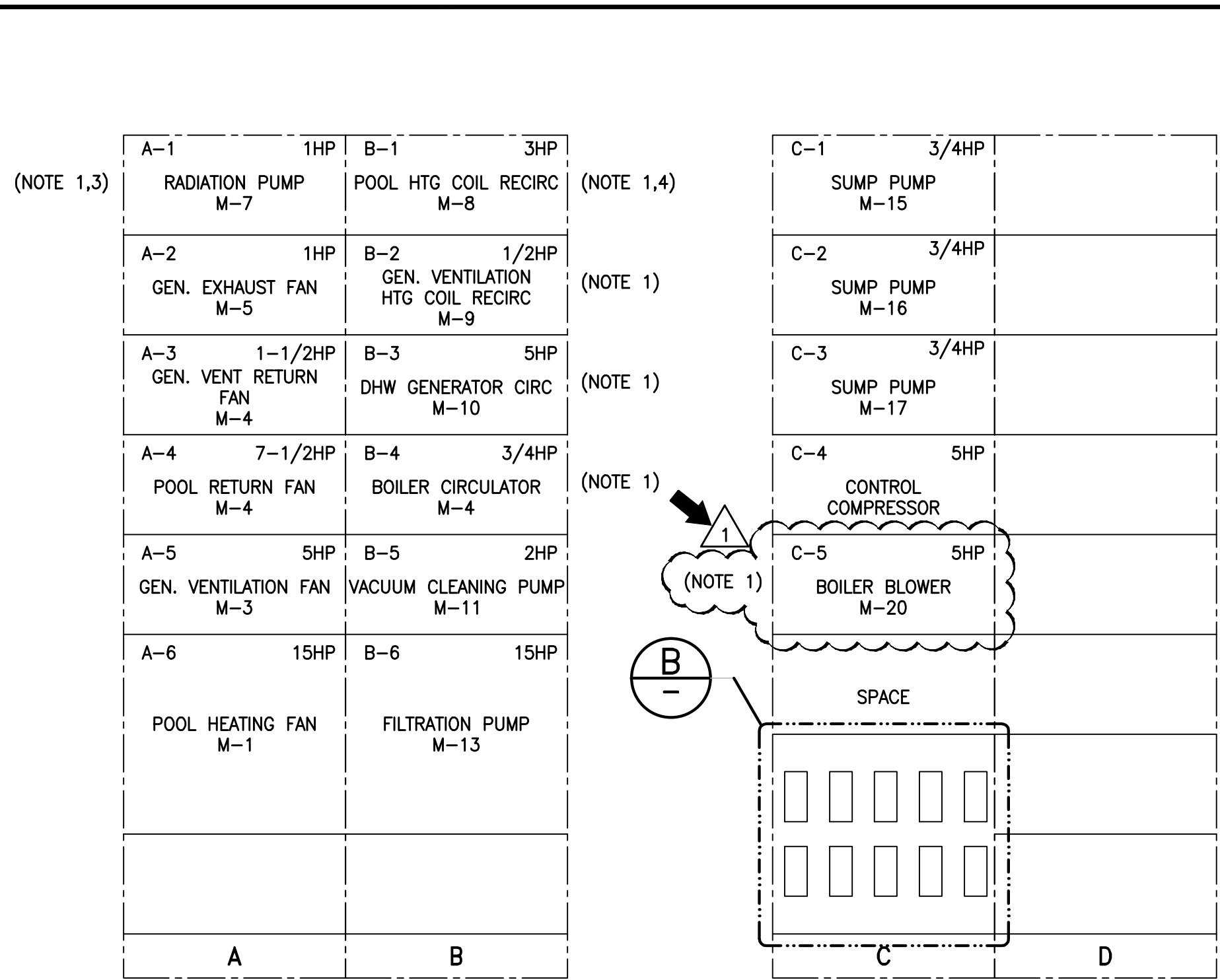
A MCC-1 ELEVATIONS SCALE: N.T.S.
