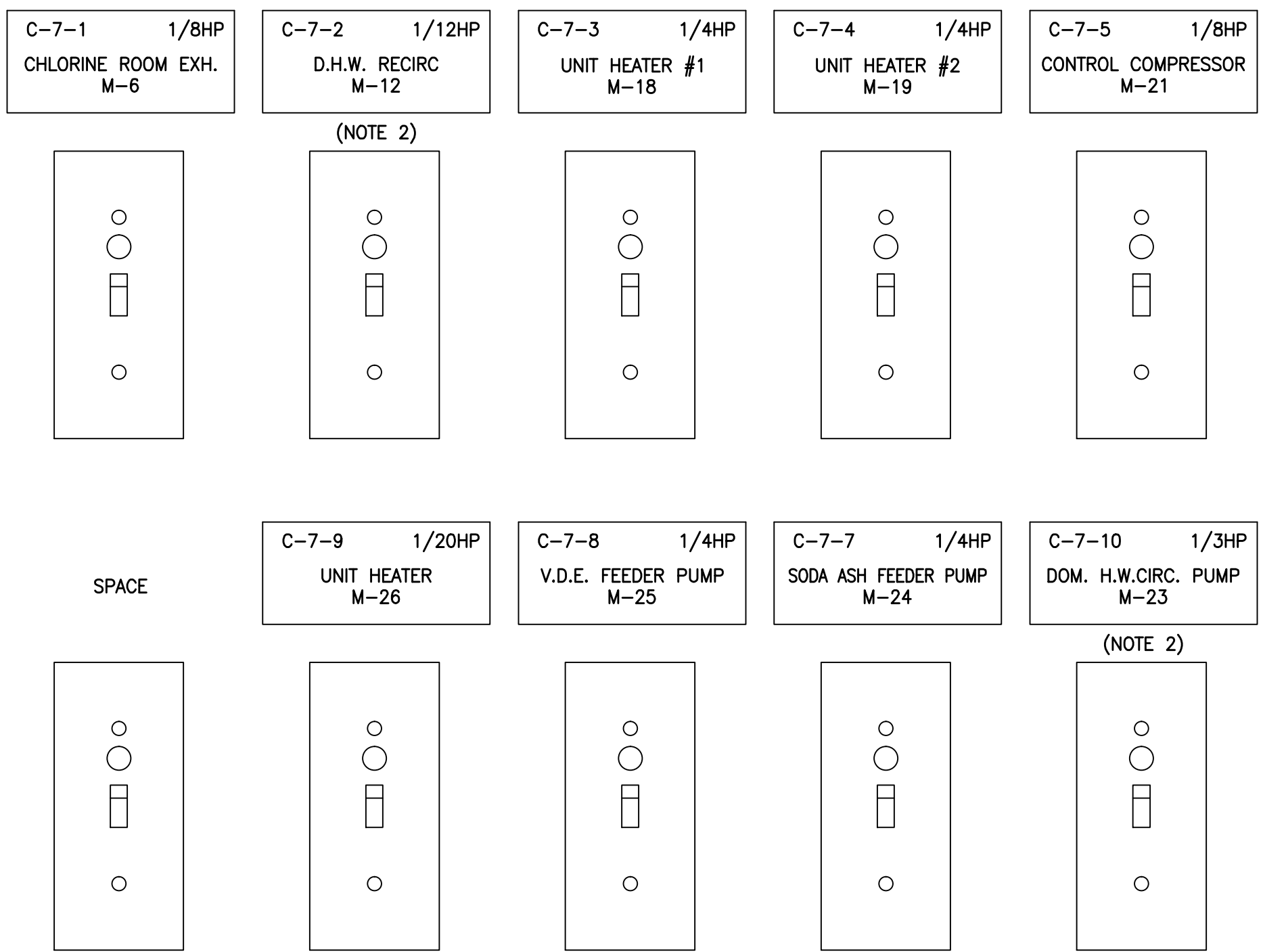
B C-7 LAYOUT SCALE: N.T.S.
