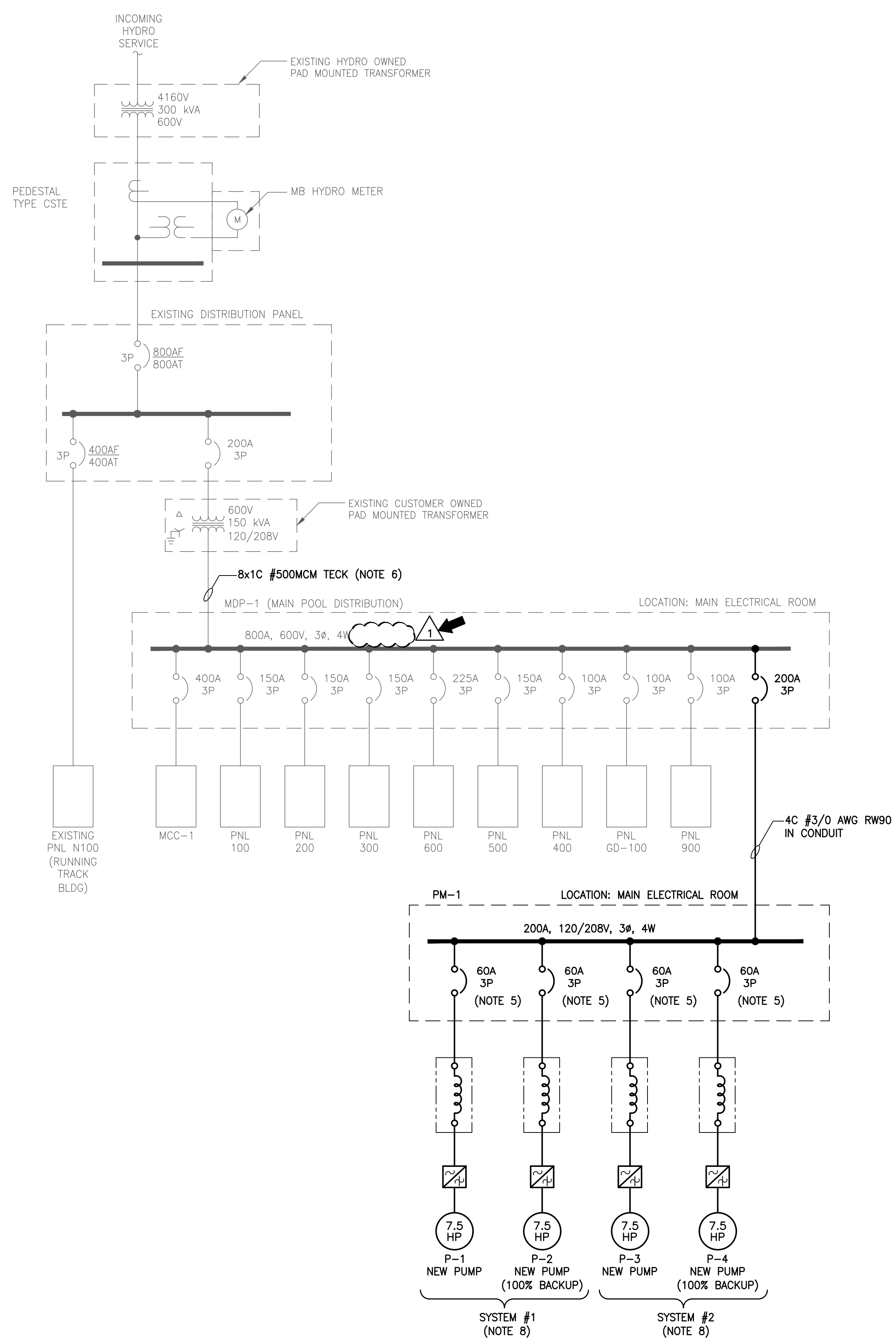
1 SINGLE LINE DIAGRAM SCALE: N.T.S.
